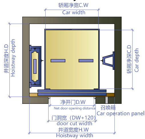
井道平面图 Hoistway width
