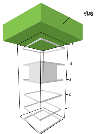
普通电梯的机房
