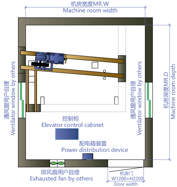
机房平面图布置图 Machine room plan
